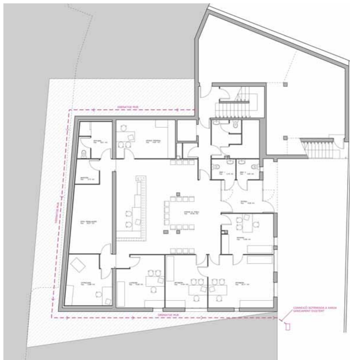
Planta de l'ambulatori
